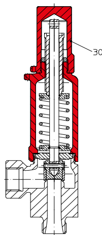
Fig. ... 963 gastight cap
